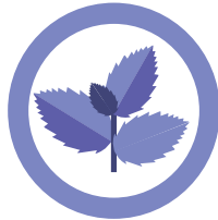
Menthol
