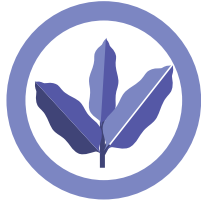
Eucalyptol
